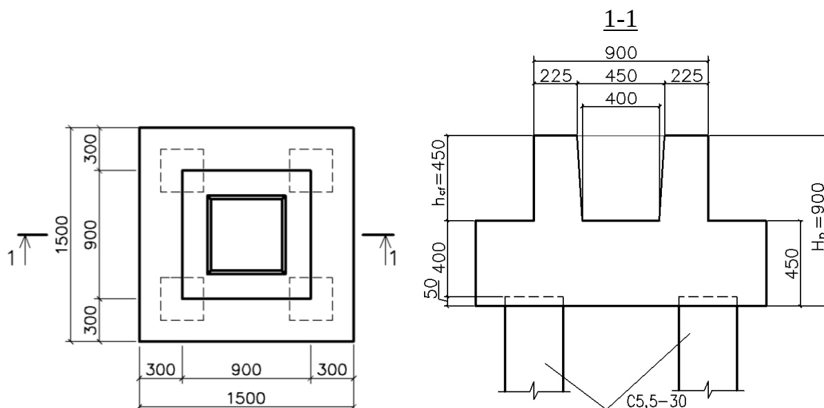
Рис. 5.2 Конструирование ростверка
