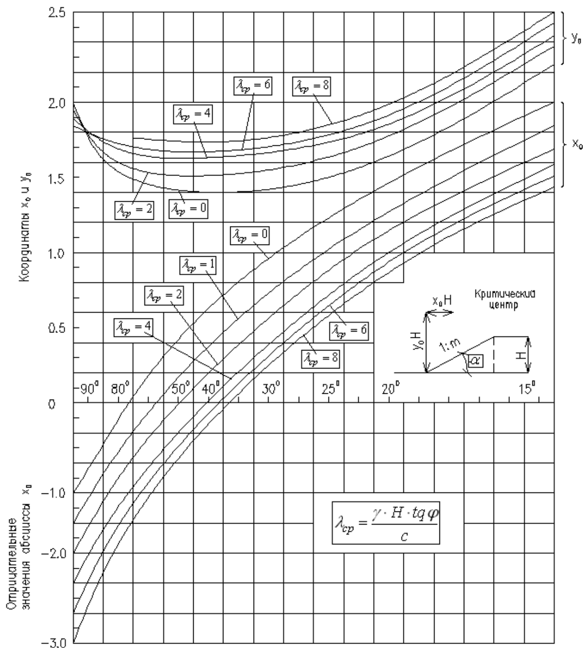
Рис. П2.1. График Ямбу для определения координат x и y центра O , наиболее опасной круглоцилиндрической поверхности скольжения с минимальным коэффициентом устойчивости K_y :
