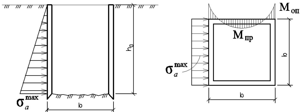
Рис. 9.2. Схема к расчету активного давления на стенки колодца и изгибающих моментов
