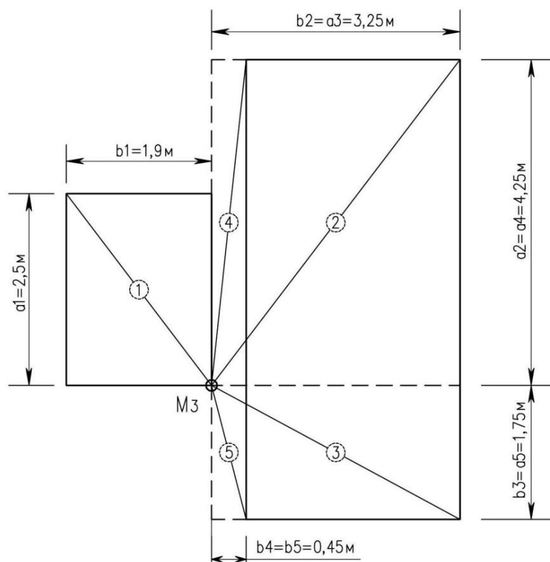
Рис.11.5. Разбивка на отдельные прямоугольники
