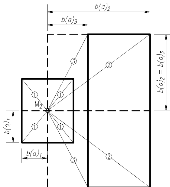
Рис.11.3. Пример разбивки прямоугольников для вертикали M_2
